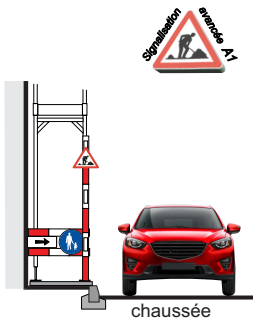
E 4 Fermeture du trottoir (déviation des piétons sur trottoir adjacent)
