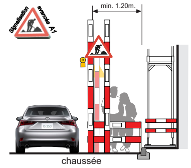
E 3 Fermeture du trottoir (déviation des piétons sur la chaussée)
